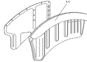
YNG040210 Guardabarros de composite para protector lateral
